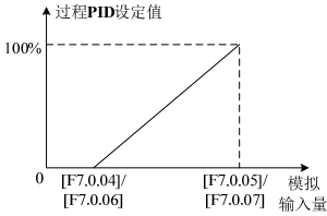
图 7-52 过程 PID 设定值定义示意图
