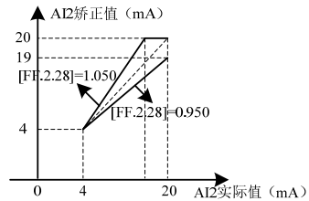
图 7-70-B AI2 增益矫正正曲线
