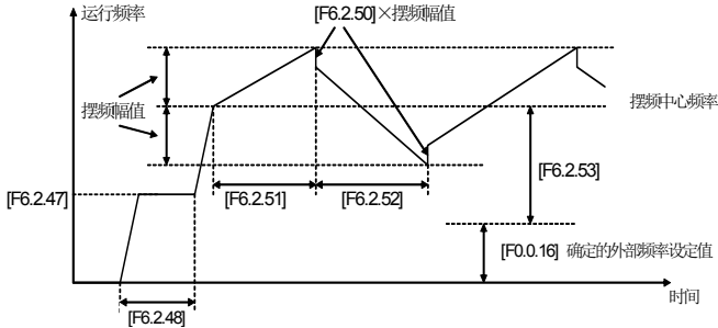
图 7-50 摆频运行示意图
