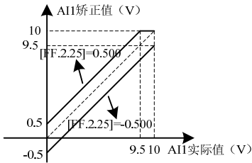
图 7-69-A AI1 零偏矫正正曲线
