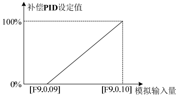
图 7-65 补偿 PID 设定值定义示意图
