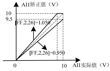
图 7-69-B AI1 增益矫正正曲线
