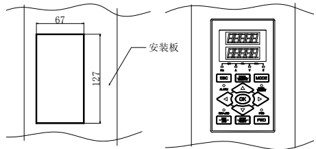
图 3-10-C 操作面板安装尺寸 3
