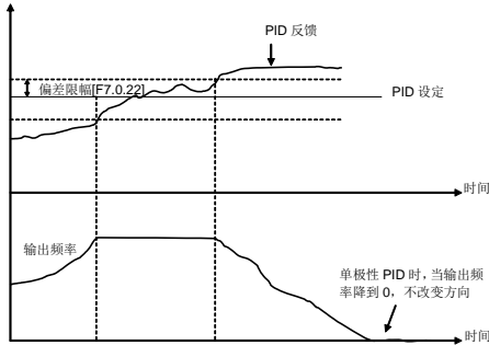
图 7-55-A 单极性 PID 控制方式
