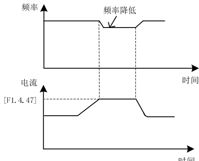
图 7-32-B 限流调节示意图
