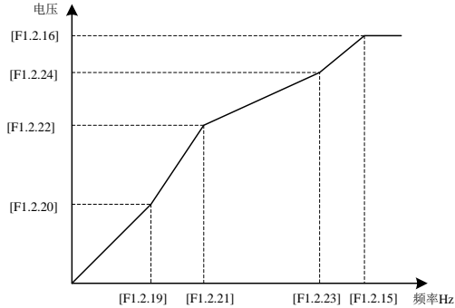
图 7-28 V/F 自定义曲线
