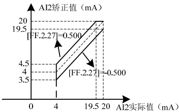
图 7-70-A AI2 零偏矫正正曲线
