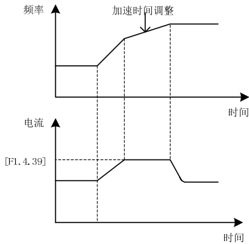
图 7-30 加/减速电流限制示意
