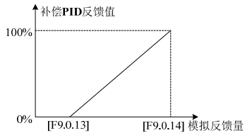
图 7-66 补偿 PID 反馈值定义示意图
