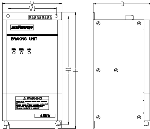
图 12-3 安装尺寸图
