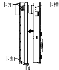
图 3-6 操作面板安装示意图
