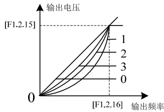
图 7-26 V/F 曲线
