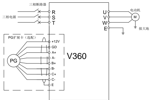
图 5-4 VC 模式运行接线
