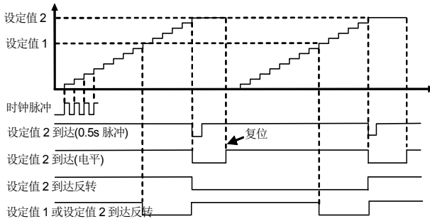
图 7-42-B 计数器功能 2
