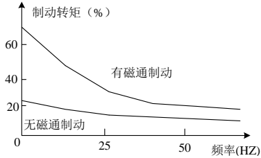
图 7-43 磁通制动曲线
