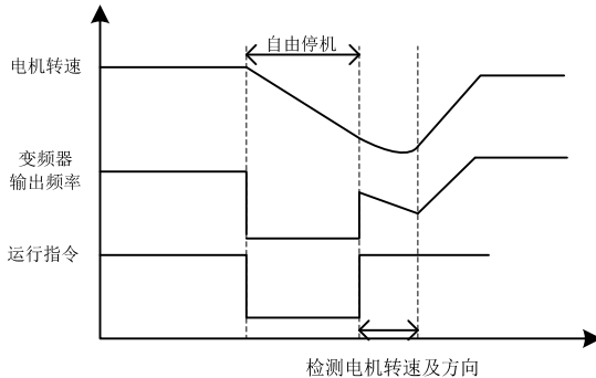
图 7-16 转速跟踪启动示意图
