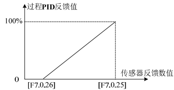
图 7-58 反馈百分比与对应传感器数值的关系曲线
