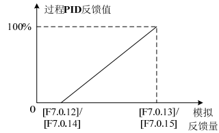
图 7-53 过程 PID 反馈值对应关系示意图
