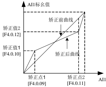
图 7-38 模拟输入 AI1 曲线
