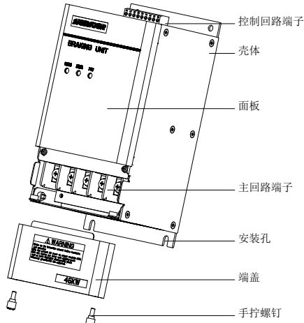
图 12-2 外观示意图
