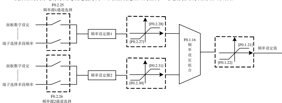
图 7-8 频率设定通道结构示意图
