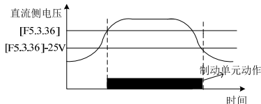
图 7-44 能耗制动
