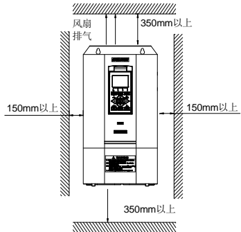
图 3-1-B 安装的间隔距离(45KW 以上)
