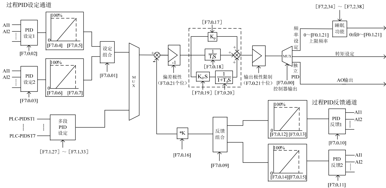
图 7-51 过程 PID 控制原理框图
