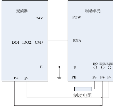
图 12-4 接线示意图
