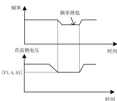
图 7-32-A 欠压调节示意图
