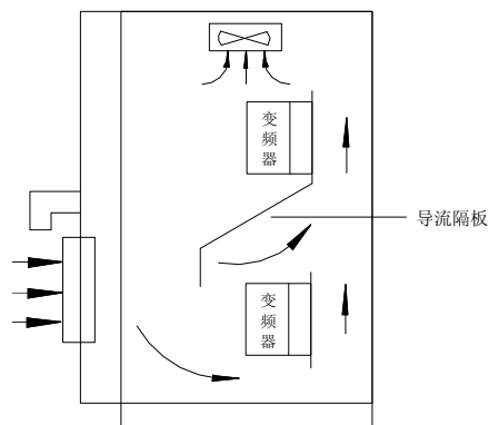
图 2-1-B 多台变频器的安装
