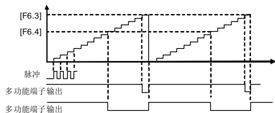
图 6-26 内部计数器功能
