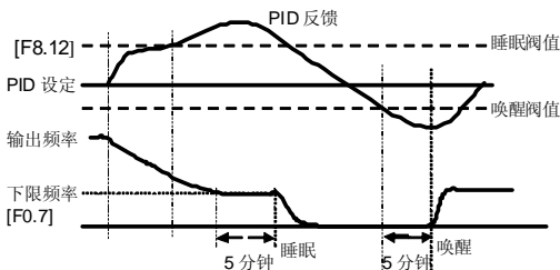
图 6-34 PID 控制的睡眠与唤醒功能
