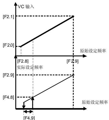
图 6-18 频率输出过零点曲线
