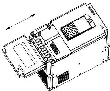
图 2-3-B 盖型盖板的拆卸与安装
