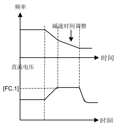
图 6-35 减速中的电压失速保护
