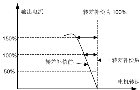
图 6-8 转差频率补偿示意图
