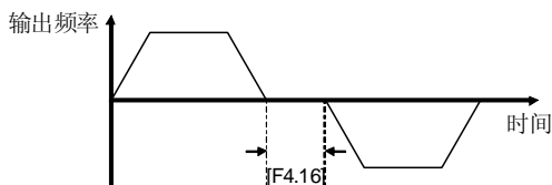
图 6-21 正反转之间的等待时间
