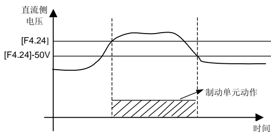
图 6-23 能耗制动
