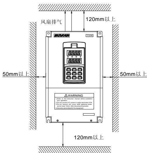
图 2-1-A 安装的间隔距离
