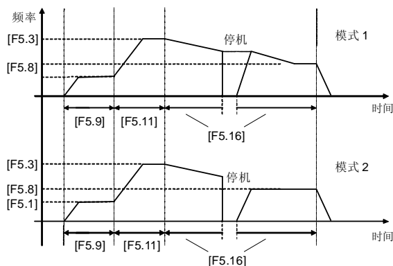
图 6-25 PLC 断点恢复
