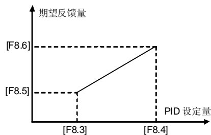
图 6-32 PID 给定量与反馈量的关系
