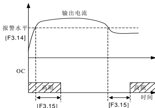
图 6-16 过载报警
