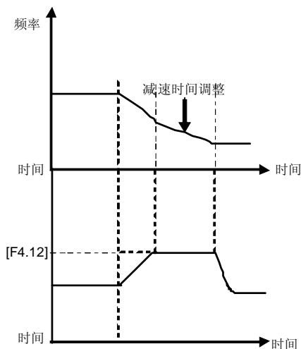
图 6-20 加速力矩与制动力矩示意图
