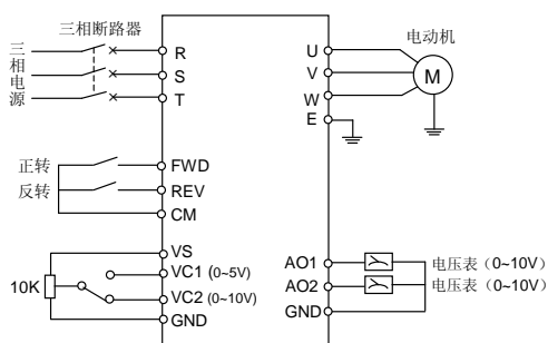
图 9-2 基本接线图
