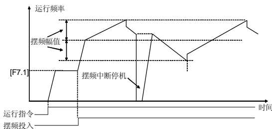
图 6-29 断点记忆恢复 (条件有效方式)
