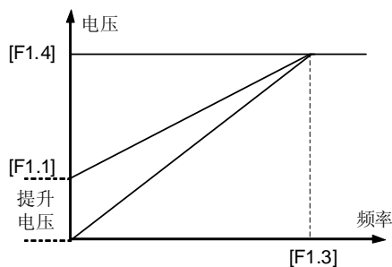
(2) 恒转矩曲线转矩提升示意图
