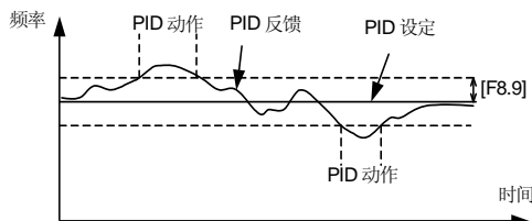
图 6-33 PID 控制允许偏差限值
