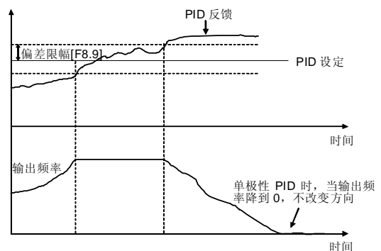
图 6-30 单极性 PID 控制方式
