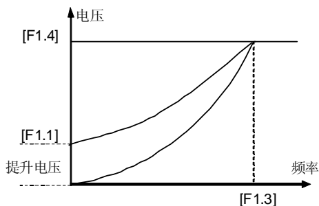
(1) 降转矩曲线转矩提升示意图
