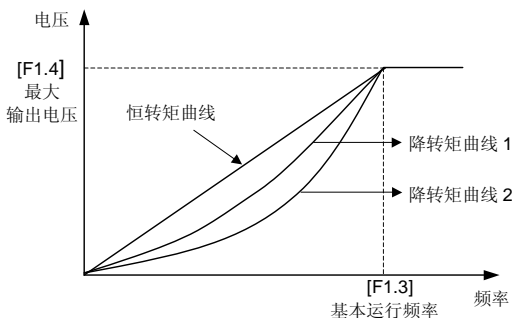
图 6-4 V/F 曲线
