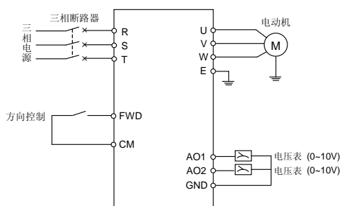
图 9-1 基本接线图
