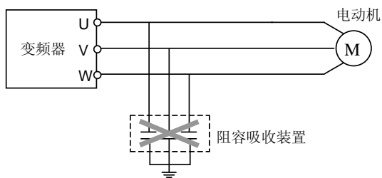
图 3-1 输出端禁止连接阻容吸收装置图
