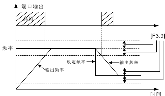
图 6-14 频率到达信号
