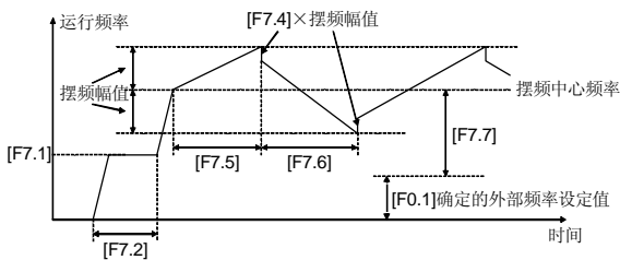
图 6-28 摆频运行过程
