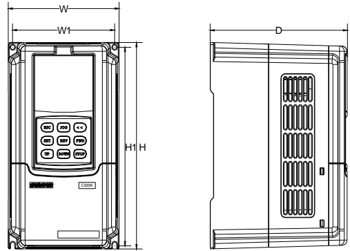
图 2-4-A 变频器安装尺寸
