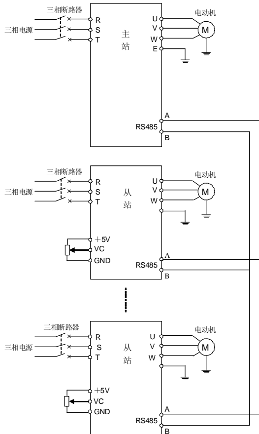
图 9-5 基本接线图
