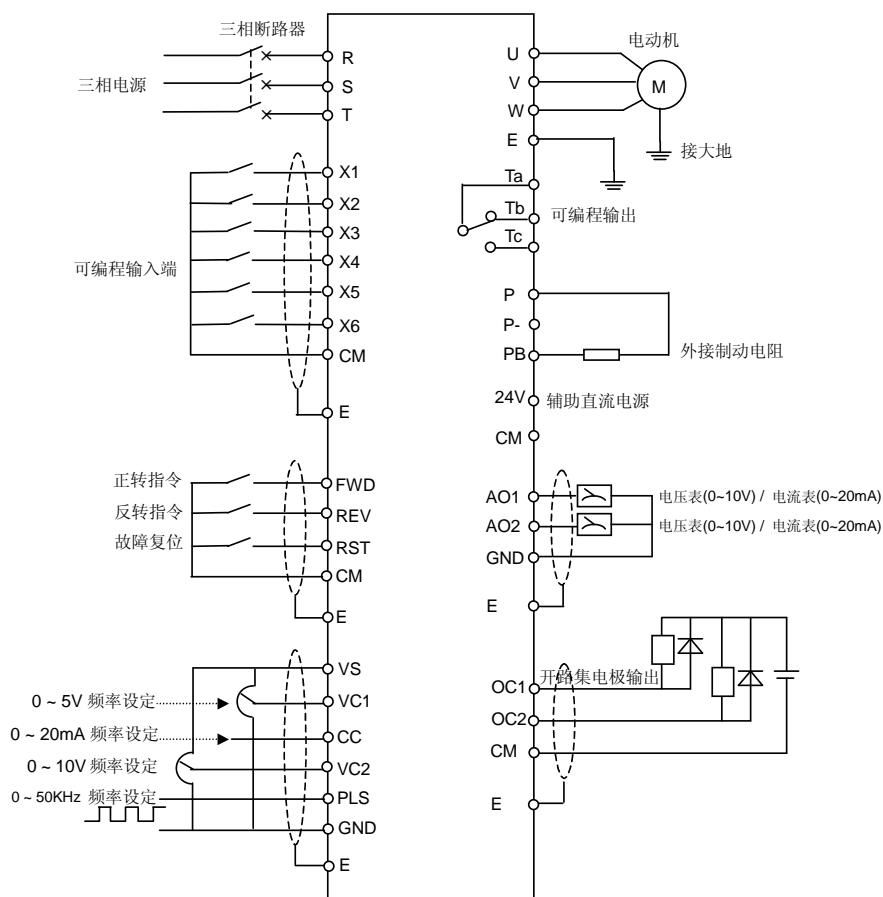
图 3-3 C320K 系列变频器基本接线图
