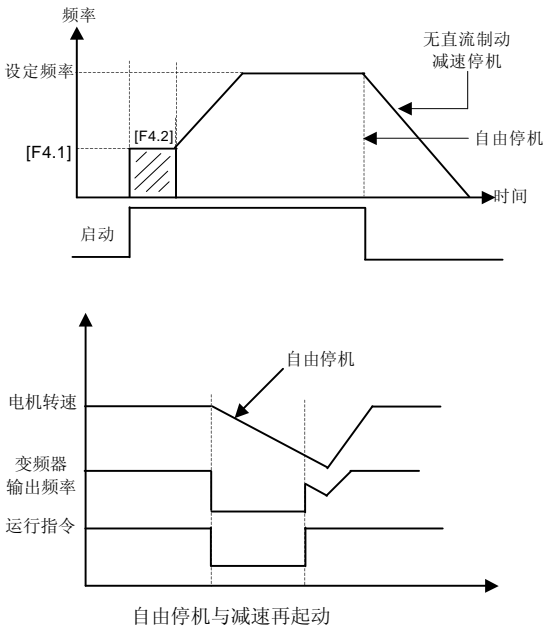
图 6-17 启动与停机频率输出曲线
