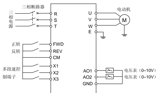
图 9-3 基本接线图
