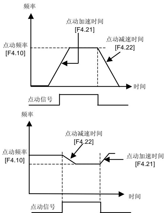
图 6-19 点动运行
