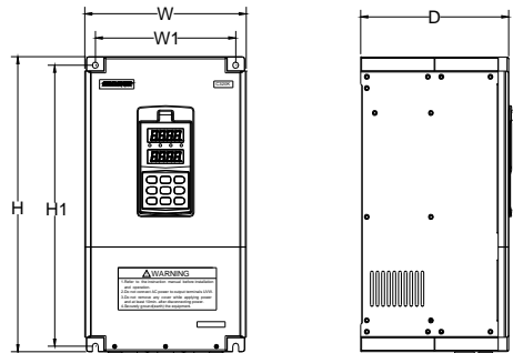
图 2-4-B 变频器安装尺寸
