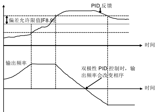
图 6-31 双极性 PID 控制方式
